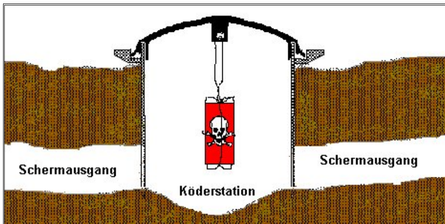
Querschnitt durch eine eingebaute Köderstation mit Köder
