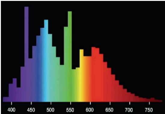
Abbildung 3: Farbspektrum/Wellenlänge [nm]: Osram T8 „Biolux“ / Osram T8 „warm-weiß“
